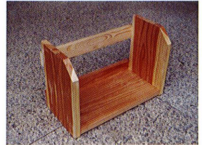
【製作する木製本立て】
